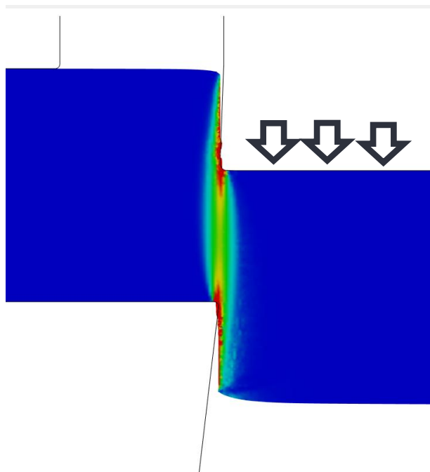
切断加工の解析
